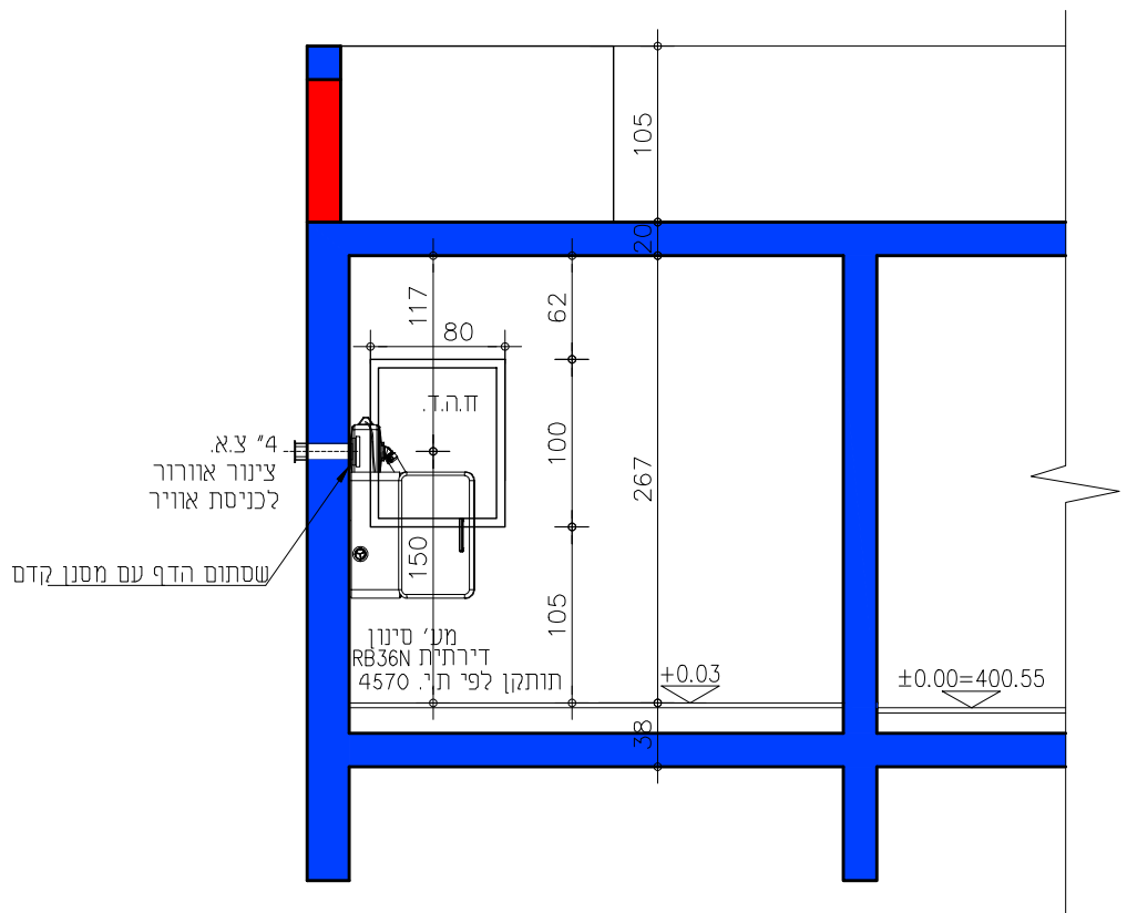
חתך E-E קנ"מ 1:50
