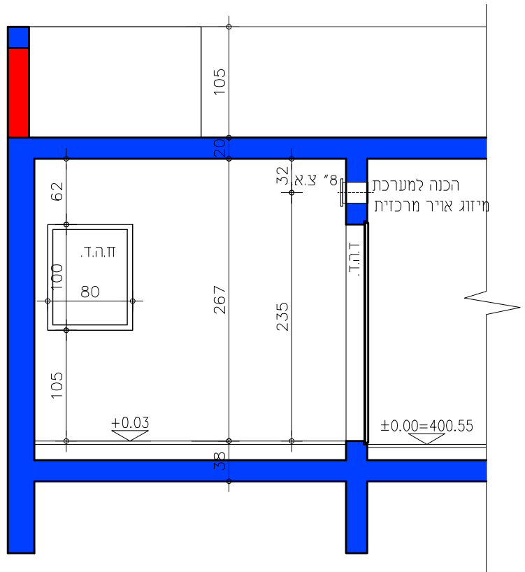
חתך G-G קנ"מ 1:50
