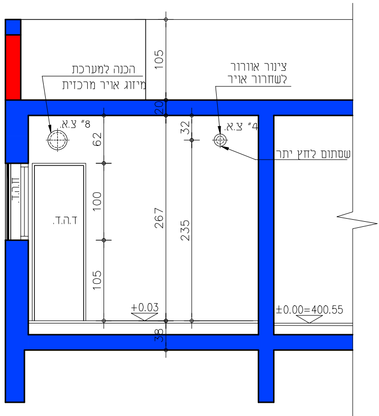
חתך S-S קנ"מ 1:50
