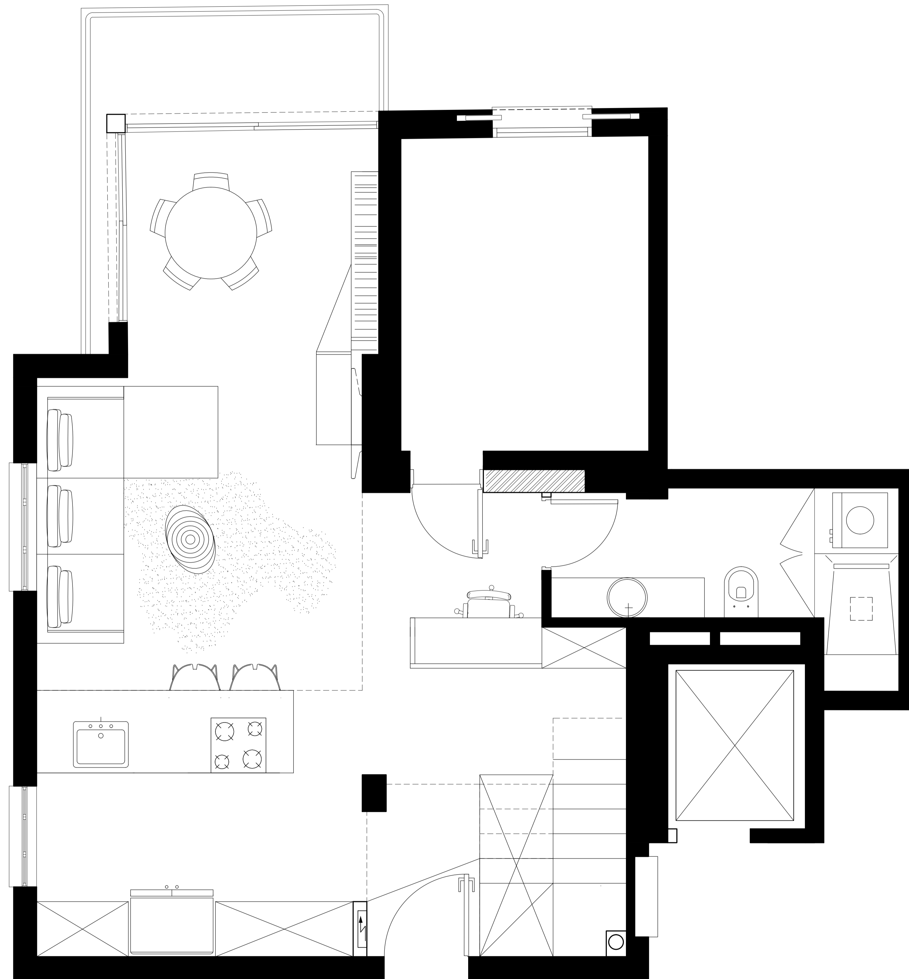
תכנית דירה במפלס 00 קומת כניסה
