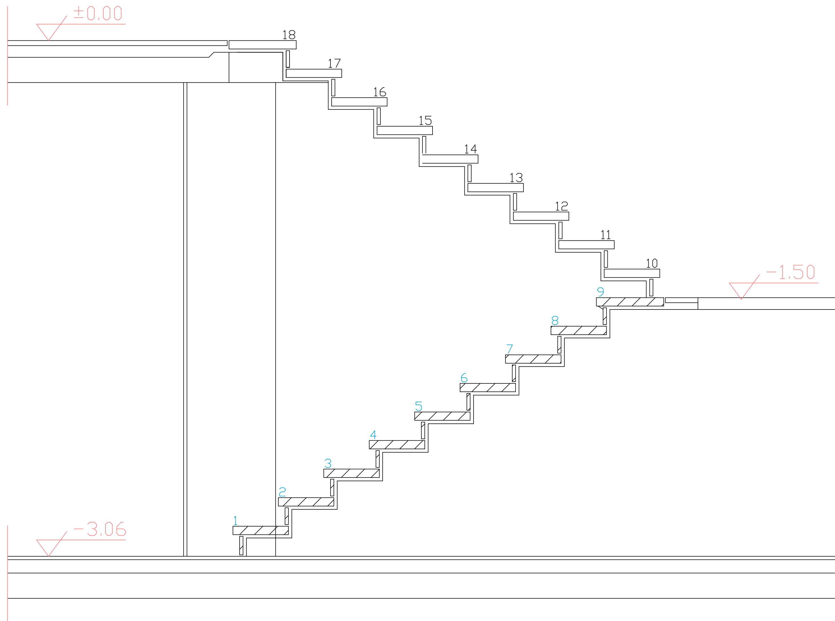
פרט מדרגות
