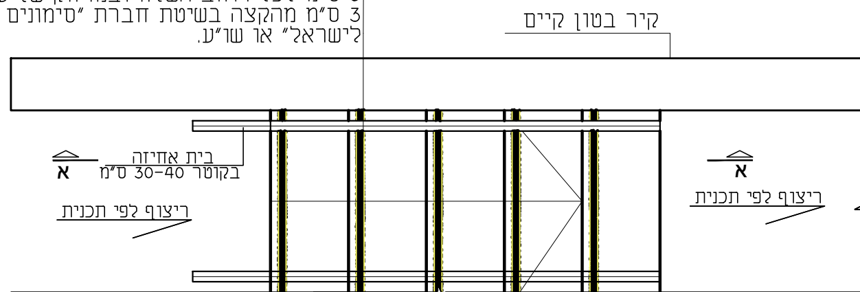
חתך אי-אי קנ"מ 1:20
