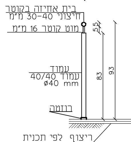
חתך בי-בי קנ"מ 1:20
