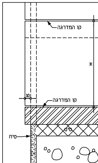
3 צד המדרגה פרט 1 : 2.5
