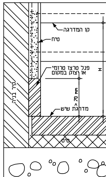
2 פנל לקיר מטייח פרט 1 : 2.5
