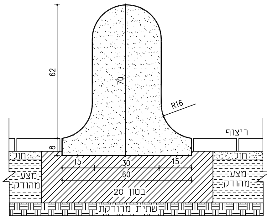
חתך
