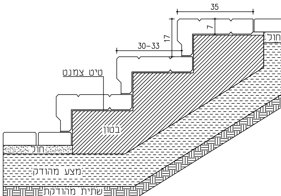
חתך מדרגות כ"א - ו ניצול מלא של גובה האלמנט
