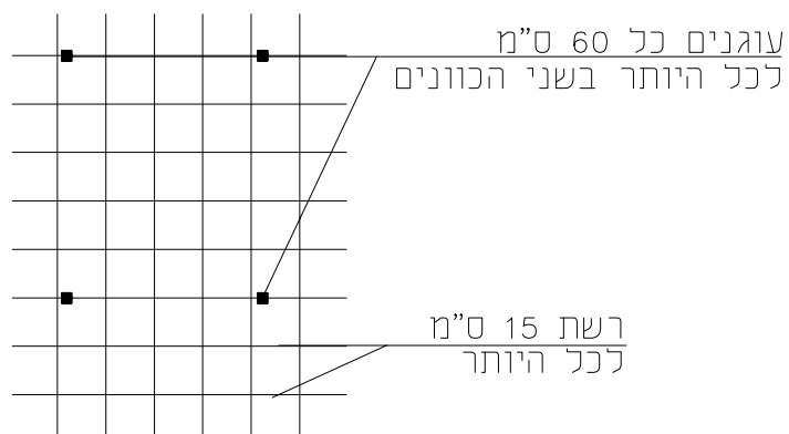
חזית סידור הרשת
