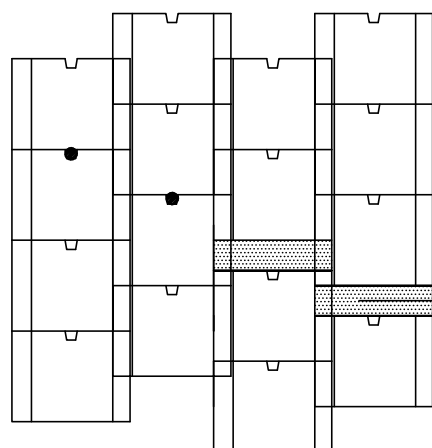
מבט על קנ"מ 1:25
