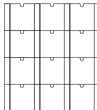
מבט על קנ"מ 1:25
