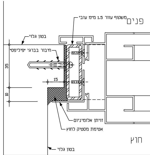
2 ב אלטרנטיבה לפרט הרכבה בטון גלוי - חוץ ופנים
