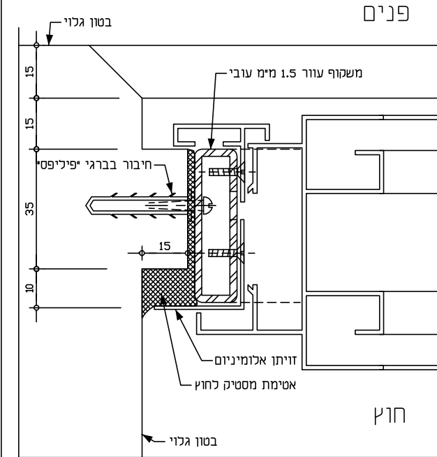
2 א אלטרנטיבה לפרט הרכבה בטון גלוי - חוץ ופנים
