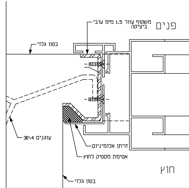
2 ג אלטרנטיבה לפרט הרכבה בטון גלוי - חוץ ופנים
