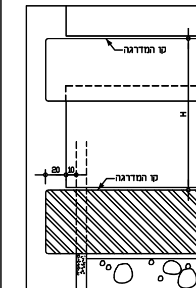
3 צד המדרגה פרט 1:2.5
