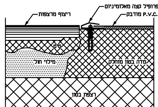
5 מעבר בין ריצוף ל-P.V.C. (ריצוף חדש)
