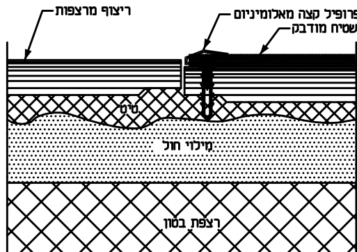
3 מעבר בין ריצוף לשטיח (ריצוף חדש)
