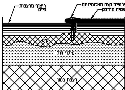
4 מעבר בין ריצוף לשטיח (ריצוף קיים)
