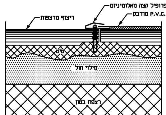
6 מעבר בין ריצוף ל-P.V.C. (ריצוף קיים)
