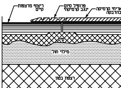
2 מעבר בין ריצוף לקרמיקה (ריצוף קיים)
