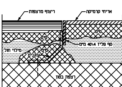
1 מעבר בין ריצוף לקרמיקה (ריצוף חדש)
