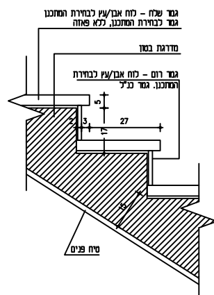
מדרגת בטון טיפוסית
