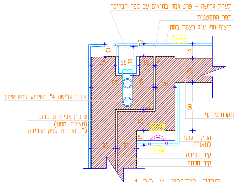
חתך מקומי X 1:20 קיר בריכה ותעלת גלישה מפגש עם קיר מרתף
