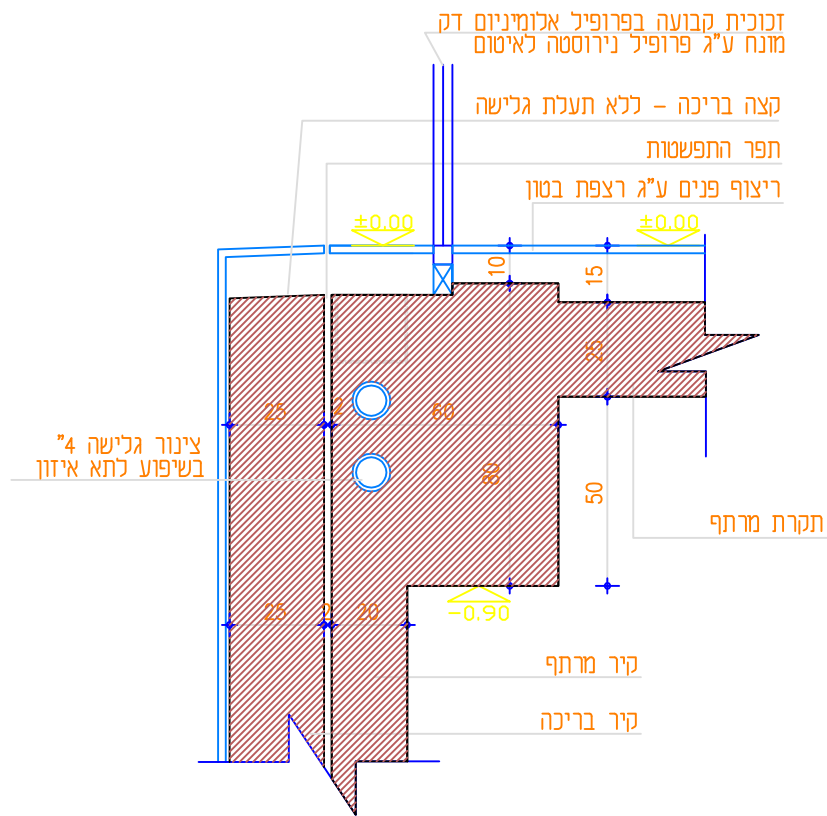
חתך מקומי Y 1:20 קיר בריכה ללא תעלת גלישה (רק אל-4)
