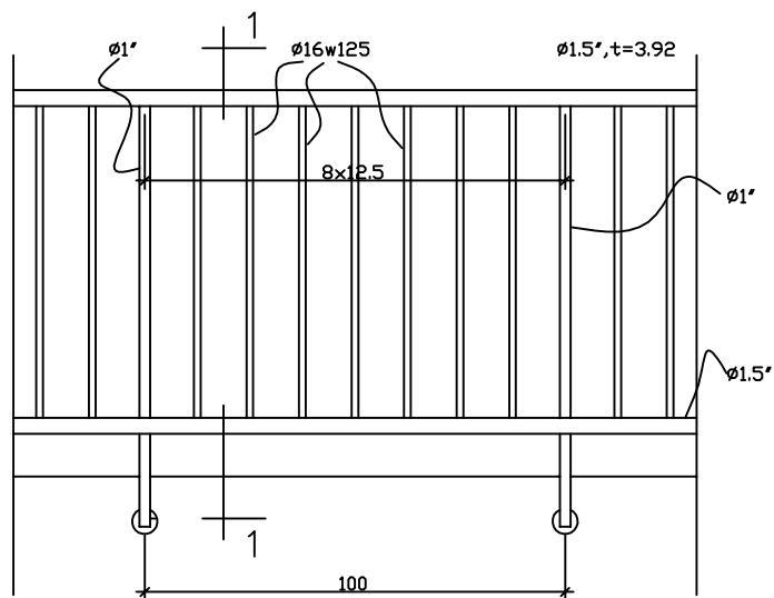
חזית המעקה 1:20
