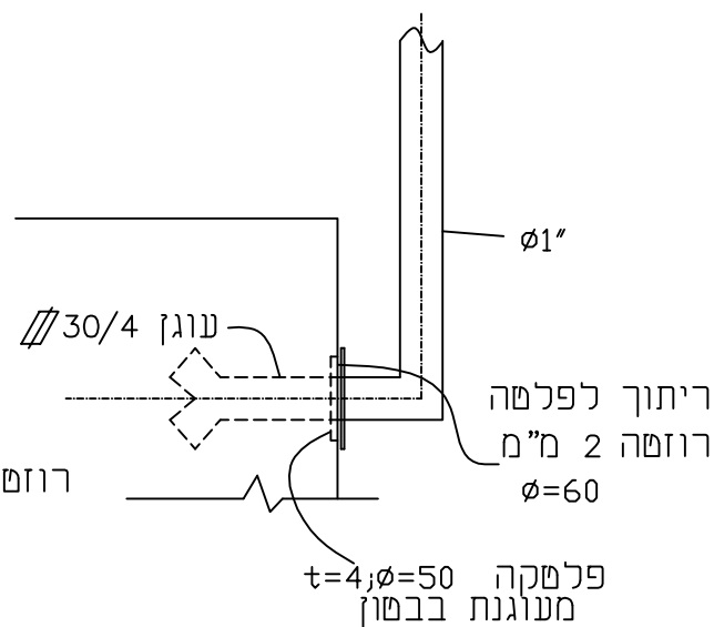
חלופה לעיגון המעקה 1:5
