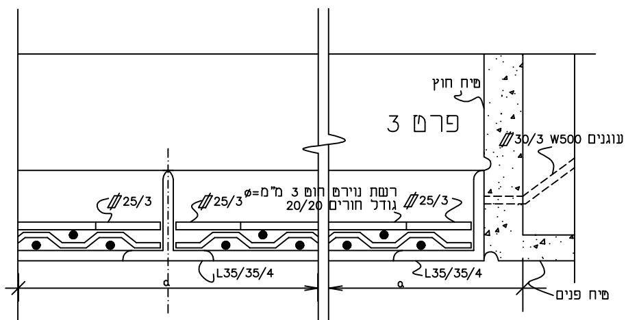
פרט חתך אפקי 1:1
