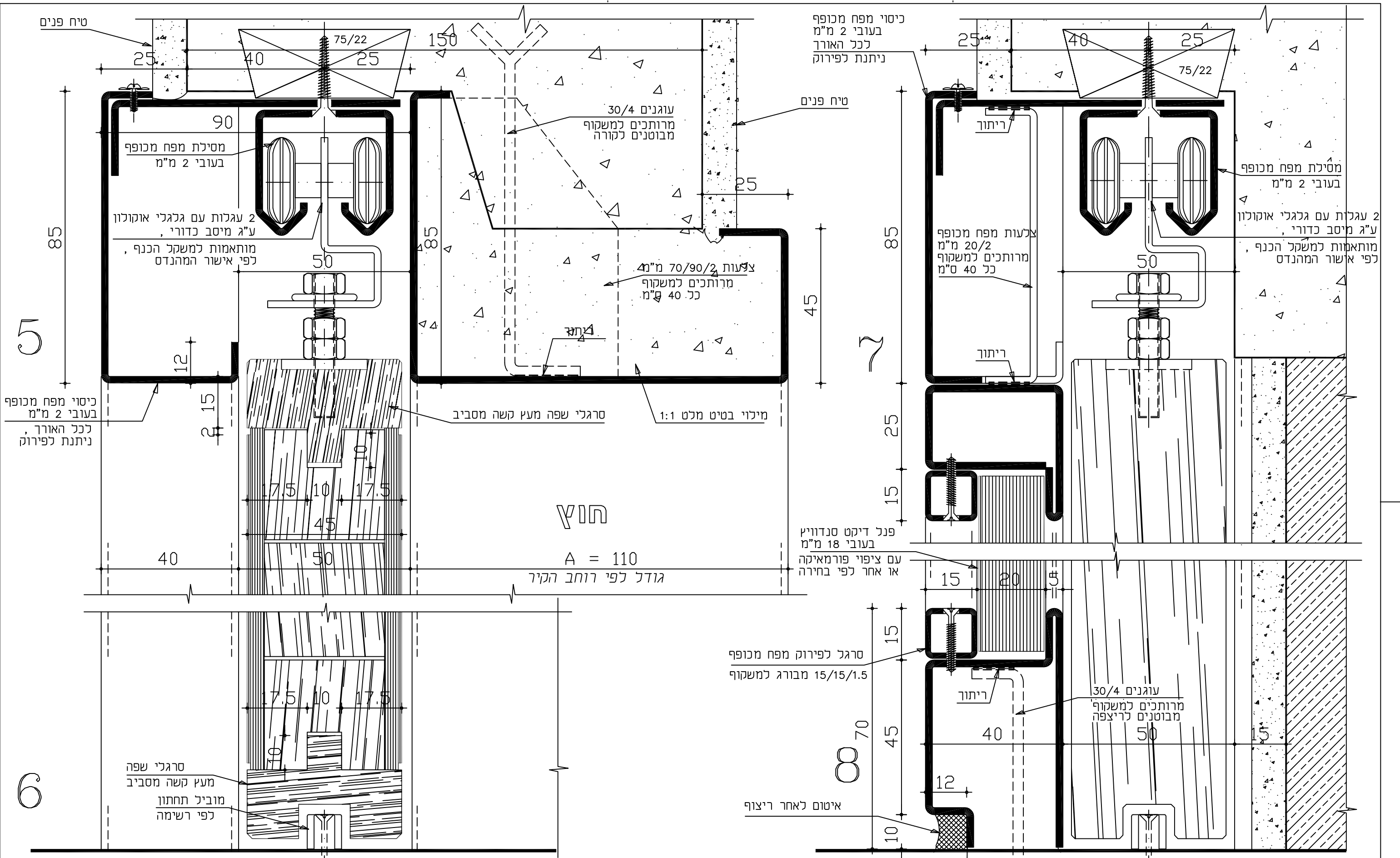
משקוף כח מכופף בולט מקו הקיר, (עובי הקיר 15 ס"מ) - כנף עץ נגררת לתוך כיס
