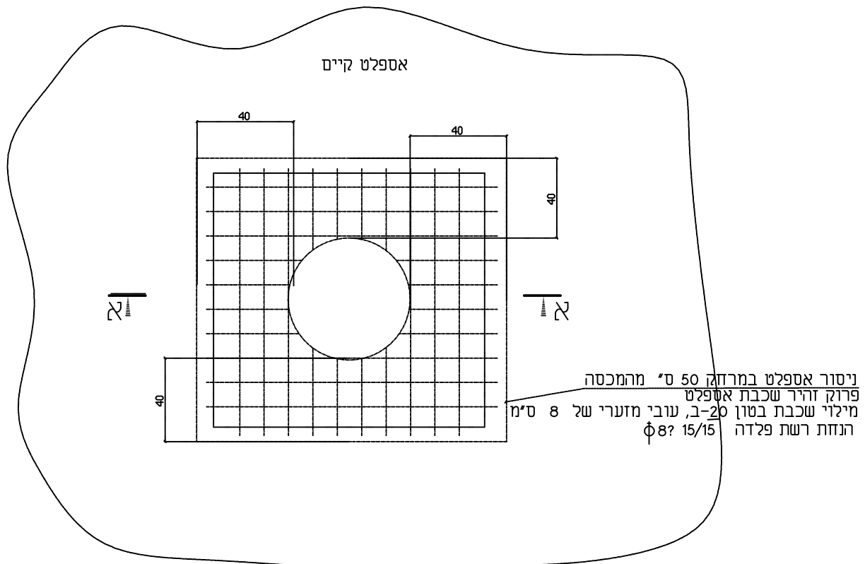
חתך ב-ב
