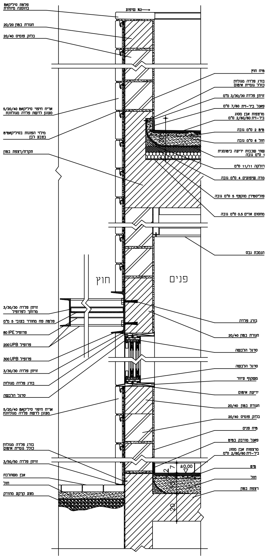
פרט חיפוי קיר במון באבן סיליקאם כולל מעקה בגג מרוצף קנ"מ 1:5
