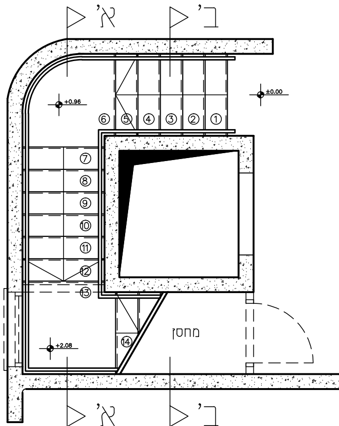
קומת כניסה קנ"מ 1:50
